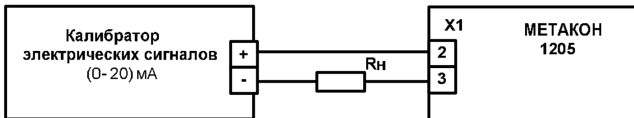
Рисунок А.6.3.1.2 – Схема подключения прибора МЕТАКОН-1205 для проведения поверки по сигналам тока
