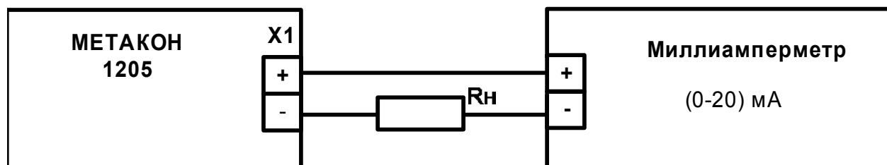
Рисунок А.6.3.3 – Схема проверки основной погрешности установления тока в токовом выходе
