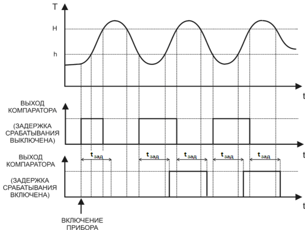
Рисунок 5 – Графики, показывающие работу компаратора с выключенной и включенной функцией задержки срабатывания
