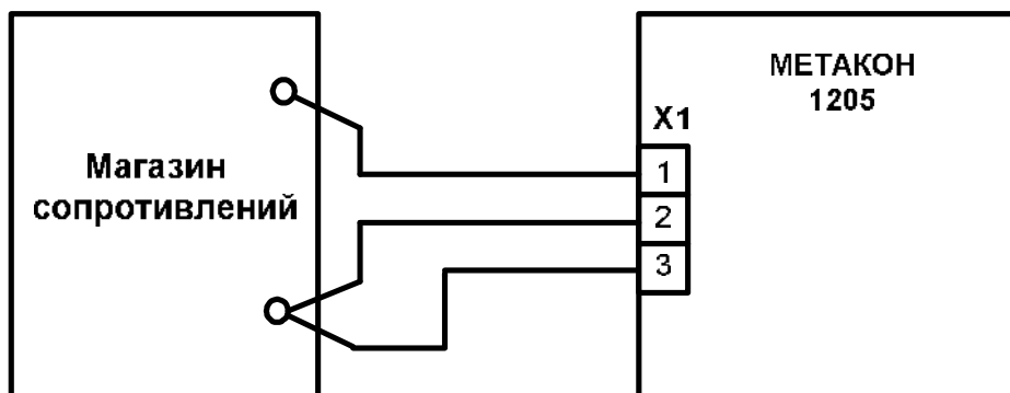
Рисунок А.6.3.1.3 – Схема подключения прибора МЕТАКОН-1205 для проведения поверки по сигналам сопротивления
