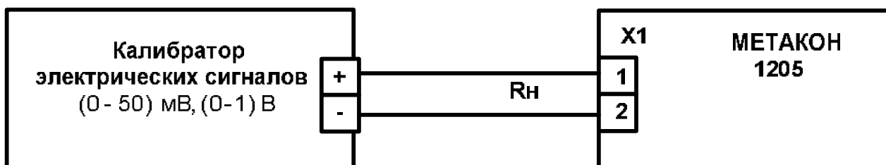
Рисунок А.6.3.1.1 – Схема подключения прибора МЕТАКОН-1205 для проведения поверки по сигналам напряжения
