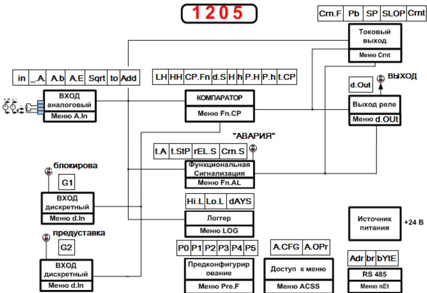
Рисунок 2 – Функциональная схема прибора МЕТАКОН-1205
