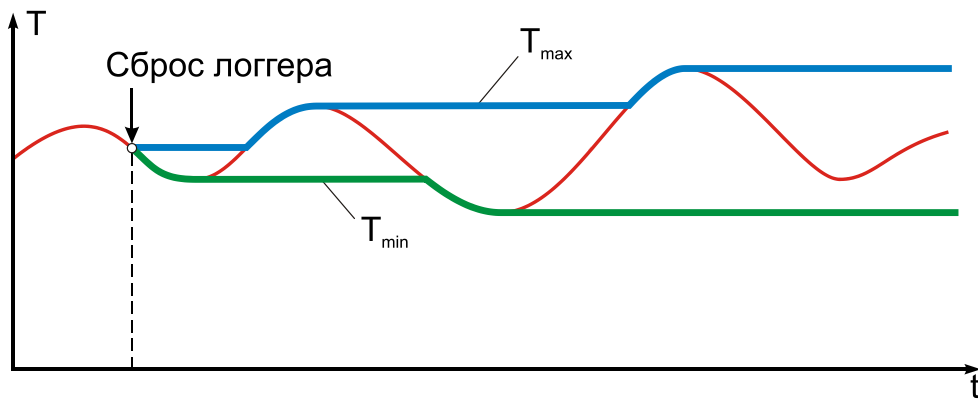
Рисунок 7 – Функция логгера прибора
