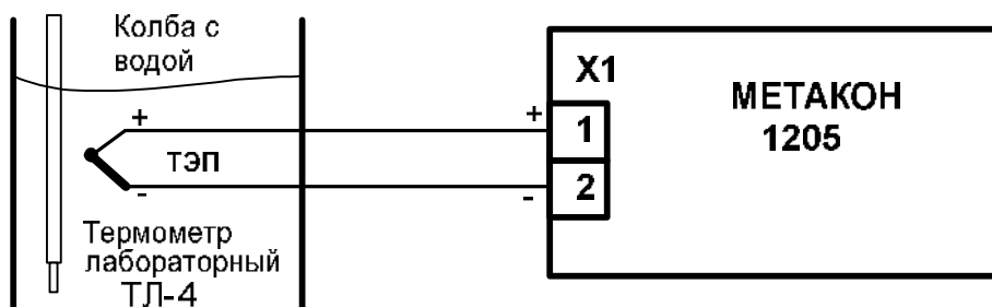
Рисунок А.6.3.2 – Схема поверки погрешности компенсации температуры холодного спая
